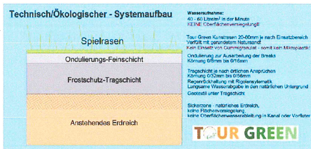
Abbildung 4: Aufbau Golfanlage
