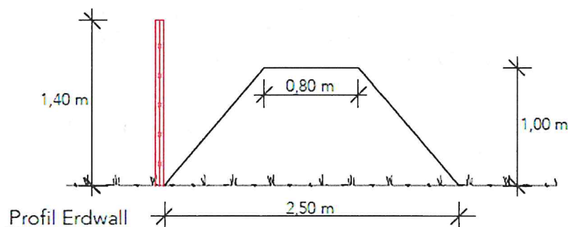
Abbildung 4: Profil Erdwall
